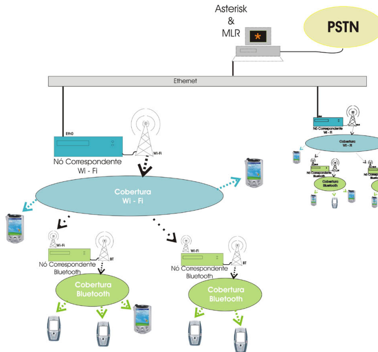
Figura 1: Arquitetura do projeto M-VoIP
