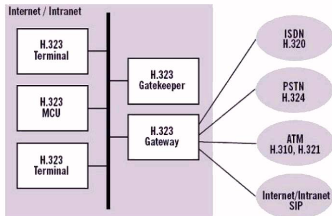
Figura 2: Elementos básicos do H.323
